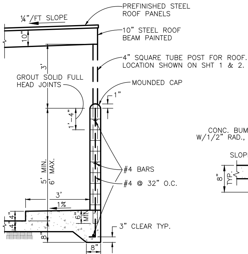
SECTION A-A
