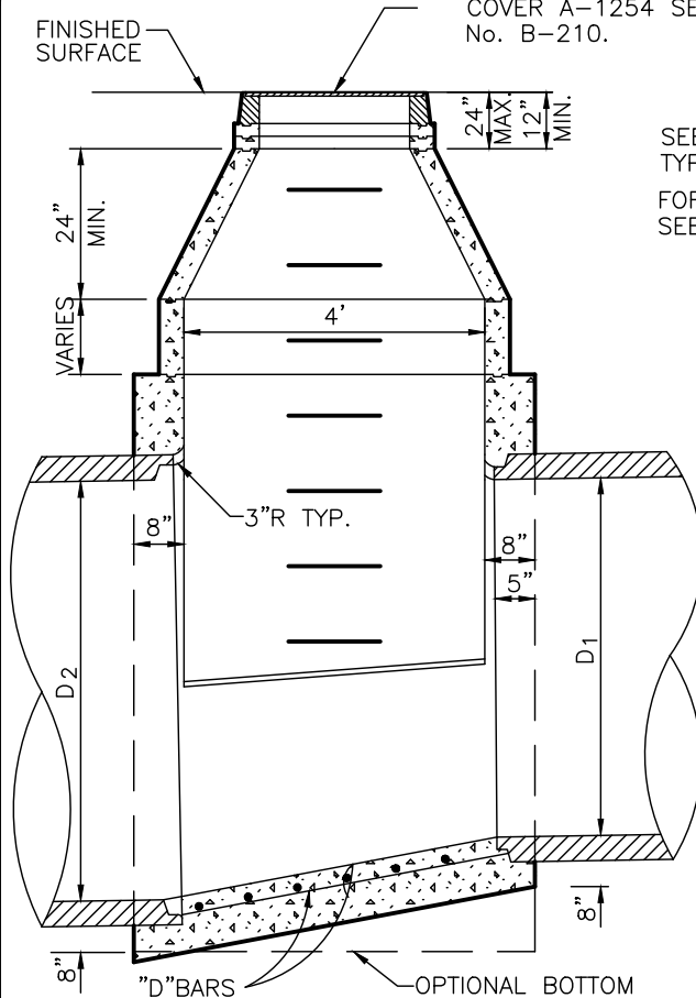
SECTION A-A
